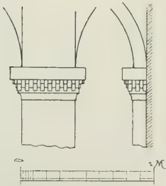
Fig. 42. Wzory słupów i pilastrów kryptowych.
